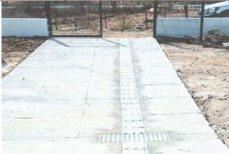
EXECUÇÃO DO PISO PODOTÁTIL EXTERNO
