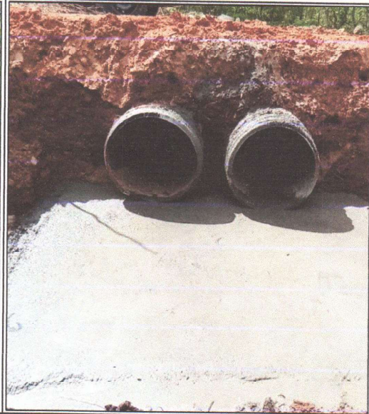
EXECUÇÃO DE BOCA DE BUEIRO DUPLO TUBULAR D= 100cm
