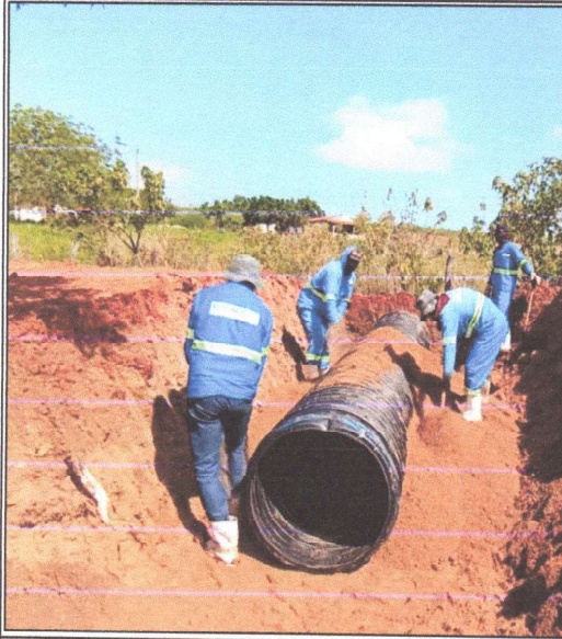
EXECUÇÃO DE CORPO DE BUEIRO SIMPLES TUBULAR D= 80cm
