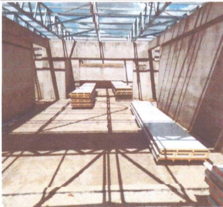
SERVIÇO DE EXECUÇÃO DE COBERTURA COM TELHA SANDUÍCHE – RECEBIMENTO DO MATERIAL.
