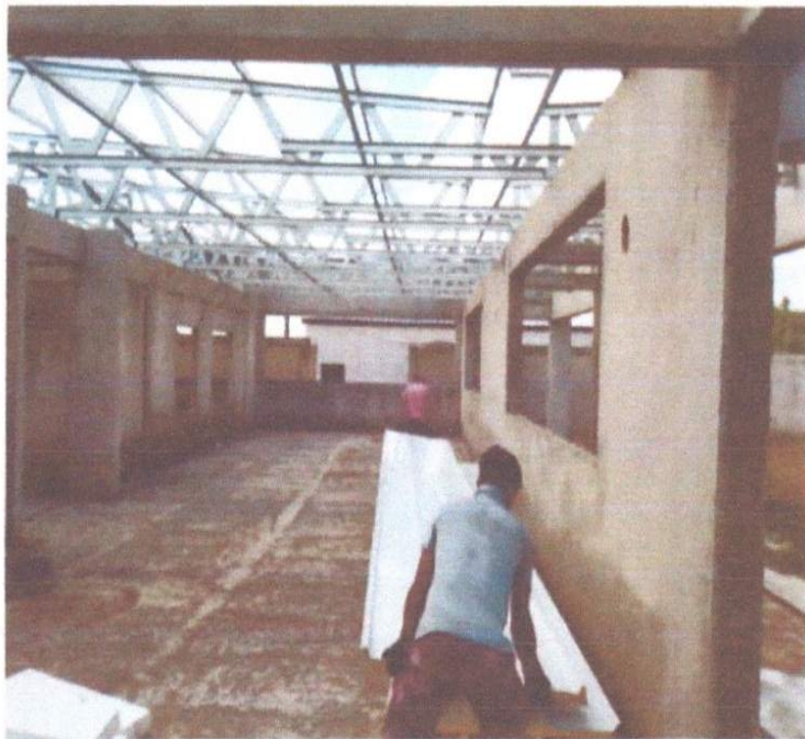
SERVIÇO DE EXECUÇÃO DE COBERTURA COM TELHA SANDUÍCHE – RECEBIMENTO DO MATERIAL.
