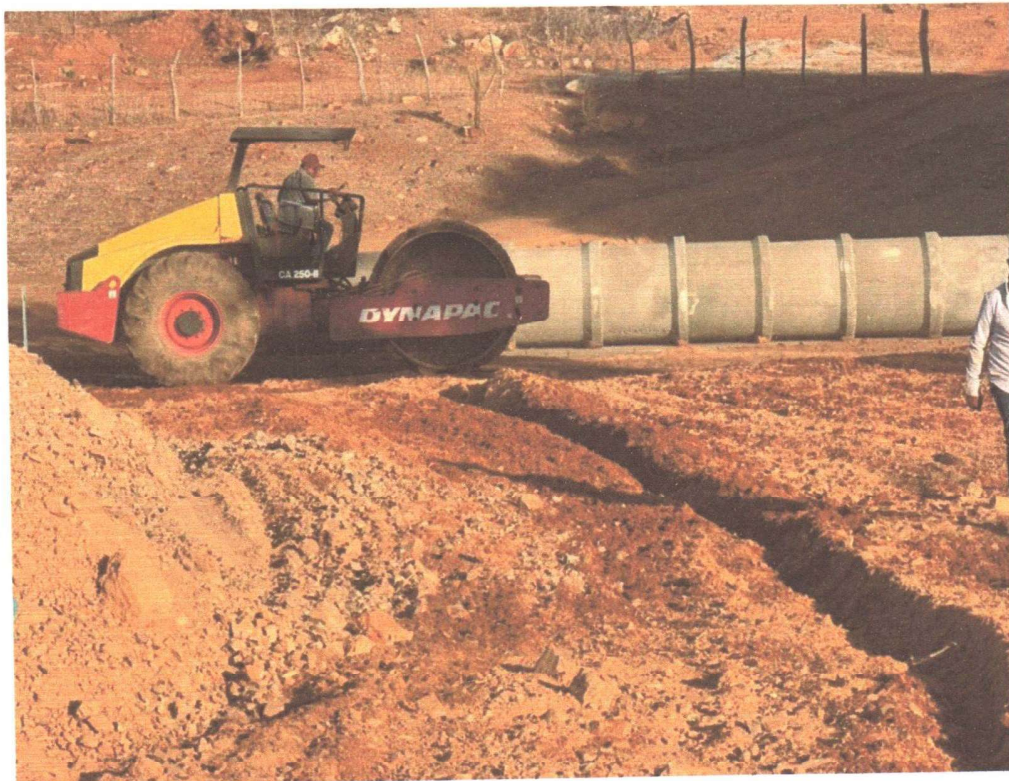
TERRAPLENAGEM
