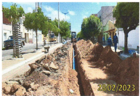
FOTO 3.34 – PANORÂMICA DAS ESCAVAÇÕES.
