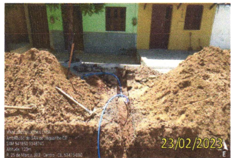
FOTO 4.6 – DETALHE DO RAMAL EM TUBO PEAD 20 mm.
