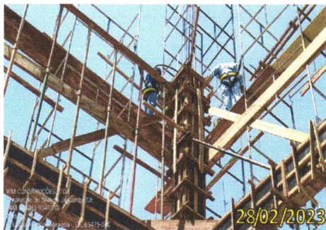
FOTO 2.3 – PANORÂMICA DA CONCRETAGEM DE PILARES.
