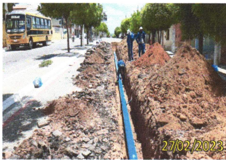
FOTO 3.33 – ASSENTAMENTO DA TUBULAÇÃO.
