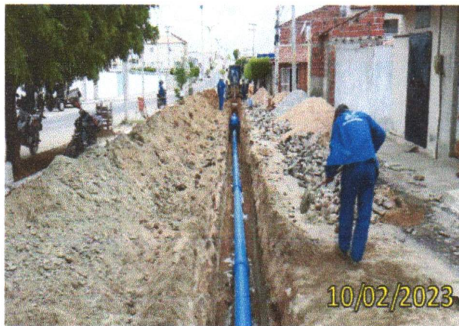
FOTO 3.7 – PANORÂMICA DAS ESCAVAÇÕES E TUBULAÇÃO ASSENTADA.
