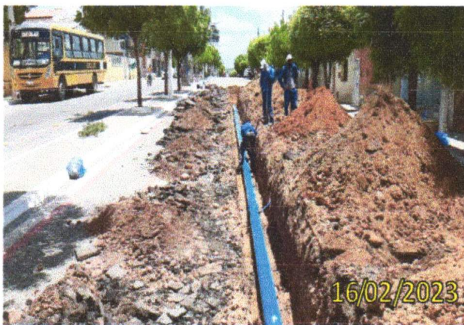
FOTO 4.3 – PANORÂMICA DA EXECUÇÃO DE LIGAÇÕES.
