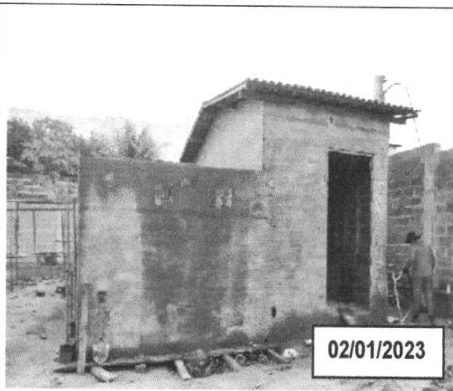
FOTO 3.7 – EXECUÇÃO DO CHAPISCO EXTERNO DO RAP DE 40 M 2 .
