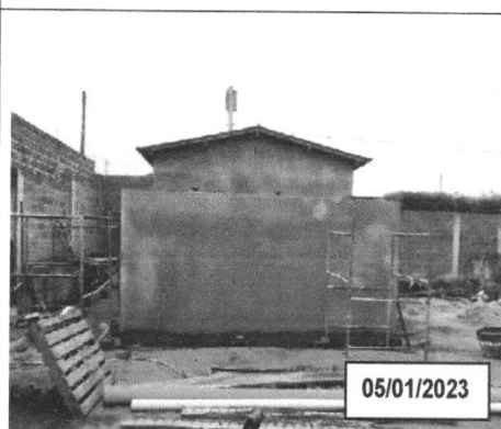
FOTO 3.6 – EXECUÇÃO DO MADEIRAMENTO DA COMBERTA DA CASA DE BOMBAS DO RAP.
