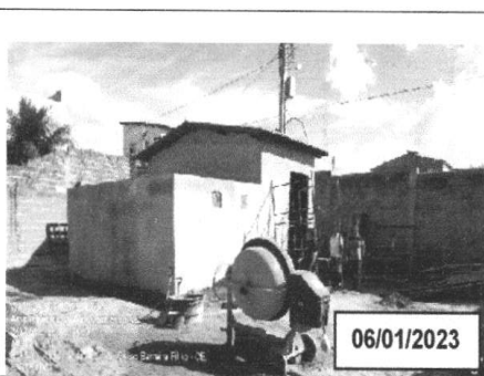
FOTO 3.9 – FINALIZAÇÃO DO REBOCO EXTERNO DO RAP DE 40 M 2 .
