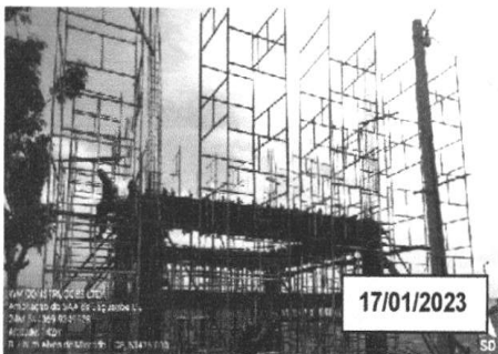
FOTO 4.25 – MONTAGEM DAS FERRAGENS DO SEGUNDO NÍVEL DOS PILARES INTERMEDIÁRIOS.
