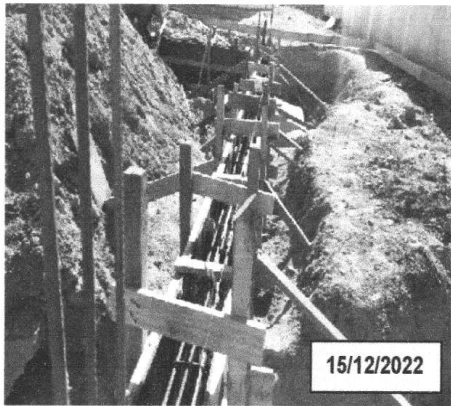
FOTO 4.9 - FORMA DA VIGA BALDRAME PRONTAS.
