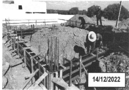
FOTO 4.8 – MONTAGEM DAS FORMAS DA VIGA BALDRAME
