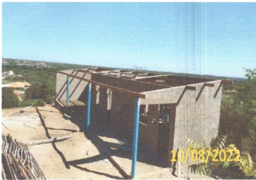
FOTO 2.5- EXECUÇÃO DA COBERTA
