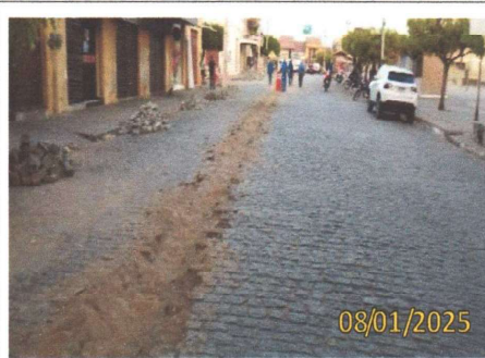
FOTO 2.1 – EXECUÇÃO DE COLCHÃO PARA ASSENTAMENTO DE PAVIMENTAÇÃO EM PARALELO.
