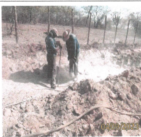
FOTO 1.31 – VISTA FRONTAL DA ESCAVAÇÃO EM MATERIAL DE 3ª CATEGORIA COM AUXÍLIO DO ROMPEDOR PNEUMÁTICO MANUAL.
