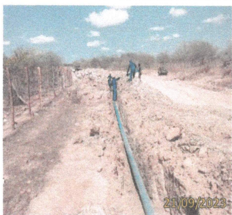
FOTO 1.47 – VISTA FRONTAL DA ESCAVAÇÃO EM MATERIAL DE 3ª CATEGORIA.
