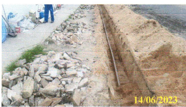
FOTO 1.15 – ASSENTAMENTO DAS TUBULAÇÕES.
