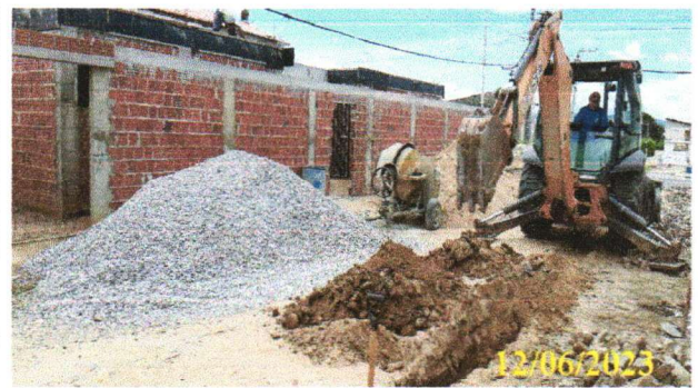
FOTO 1.12 – ESCAVAÇÃO DA VALA COM AUXÍLIO DE RETROESCAVADEIRA.
