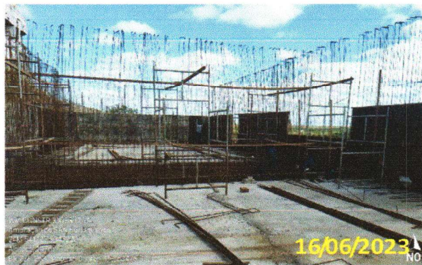
FOTO 3.9 – VISTA FRONTAL DAS FERRAGENS DA PAREDE DIVISÓRIA DO POÇO DE SUÇÃO.
