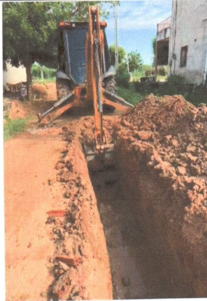
ESCAVAÇÃO MECANIZADA DE VALA
