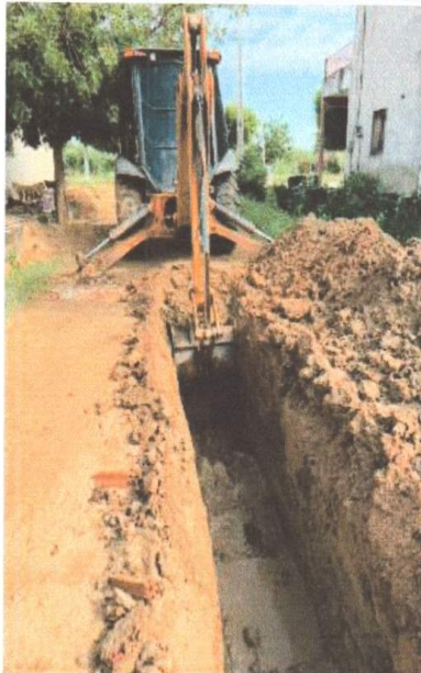
ESCAVAÇÃO DE VALA E SINALIZAÇÃO DE OBRA
