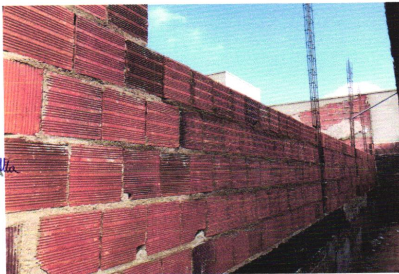
FOTO – 10 – EXECUÇÃO DE ESTRUTURAS, ALVENARIA DE EMBASAMENTO, ALVENARIAS DE FECHAMENTO E IMPERMEABILIZAÇÃO DE VIGA BALDRAME
