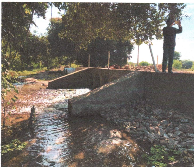
FOTO – 06 – ALVENARIA DE PEDRA – (DATA 09/11/2022 A 17/11/2022 E 05/12/2022 A 23/12/2022)
