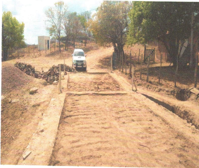
FOTO – 09 - ATERRO COMPACTADO – (DATA 21/10/2022 A 31/10/2022)
