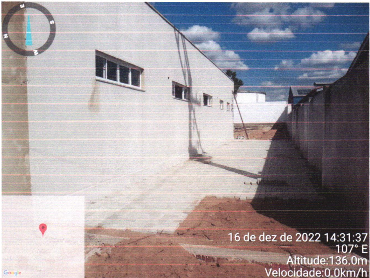
FOTO – 01 – (PISOS EXTERNOS E URBANIZAÇÃO) NA ÁREA DE SECAGEM DE ROUPA) - LASTRO DE AREIA, PISO INTERTRAVADO TIPO TIJOLINHO (19,9x10x4)cm NA COR CINZA
