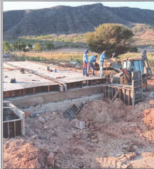
CONCRETAGEM DE VIGAS
