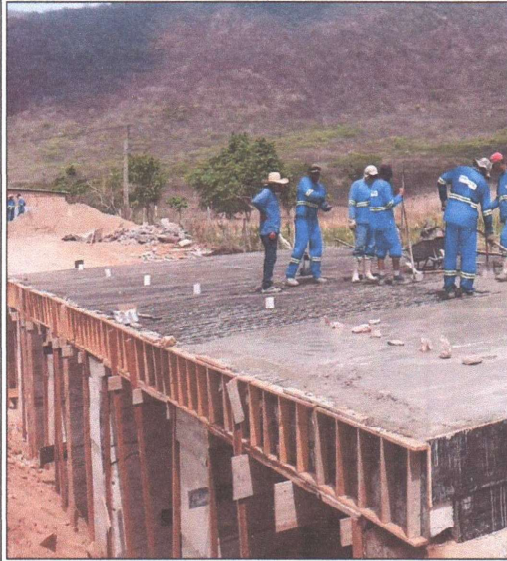
CONCRETAGEM DE LAJE
