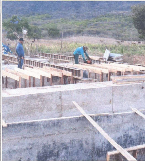
FABRICAÇÃO DE FÔRMA PARA VIGAS
