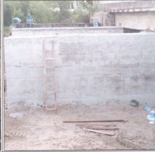
EXECUÇÃO DE ALVENARIA EM PEDRA ARGAMASSADA
