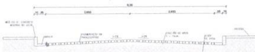
4 SEÇÃO TIPO 2 RUA OTÍLIA DIÓGENES 1:200
