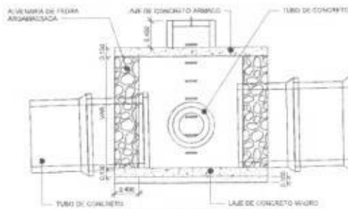
4 CORTE POÇO DE VISITA 1 : 30
