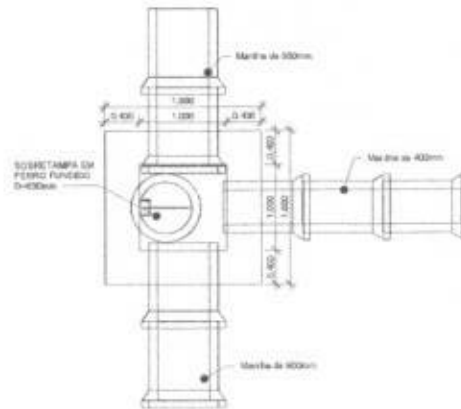
2 PLANTA P.V. TIPO 1 1 : 30
