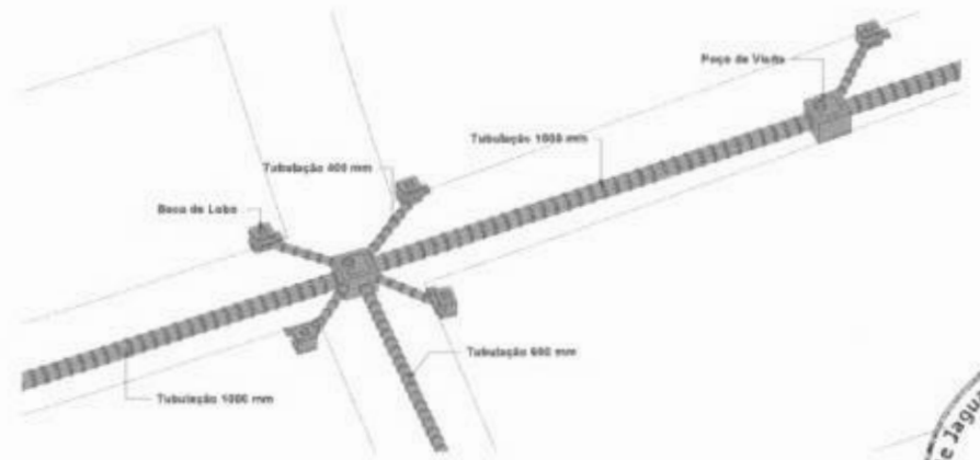
2 PERSPECTIVA DA REDE DE DRENAGEM
