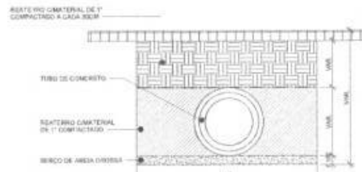
5 DETALHE DAS VALAS 1 : 30
