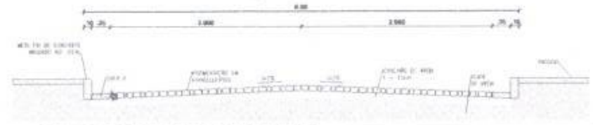
6 SEÇÃO TIPO 2 FRANCISCO LIMA SILVEIRA 1:200
