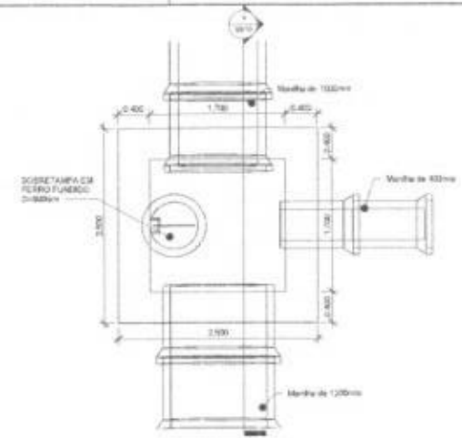
3 PLANTA P.V. TIPO 2 1 : 30
