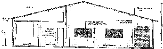
03 CORTE A-A ESCALA 1:100
