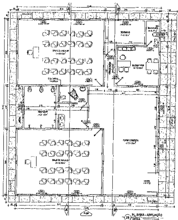
01 PLANTA - AMPLIACAO ESCALA 1:100
