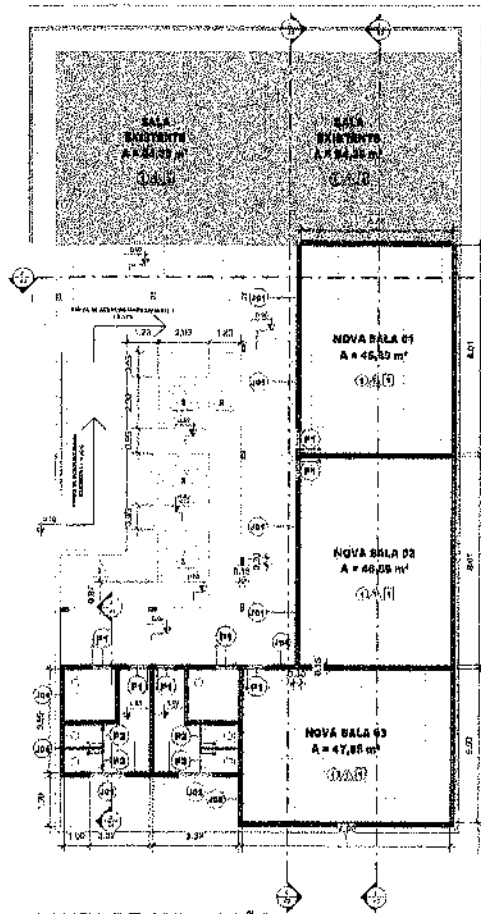
2 PLANTA DE AMPLIAÇÃO 1:100
