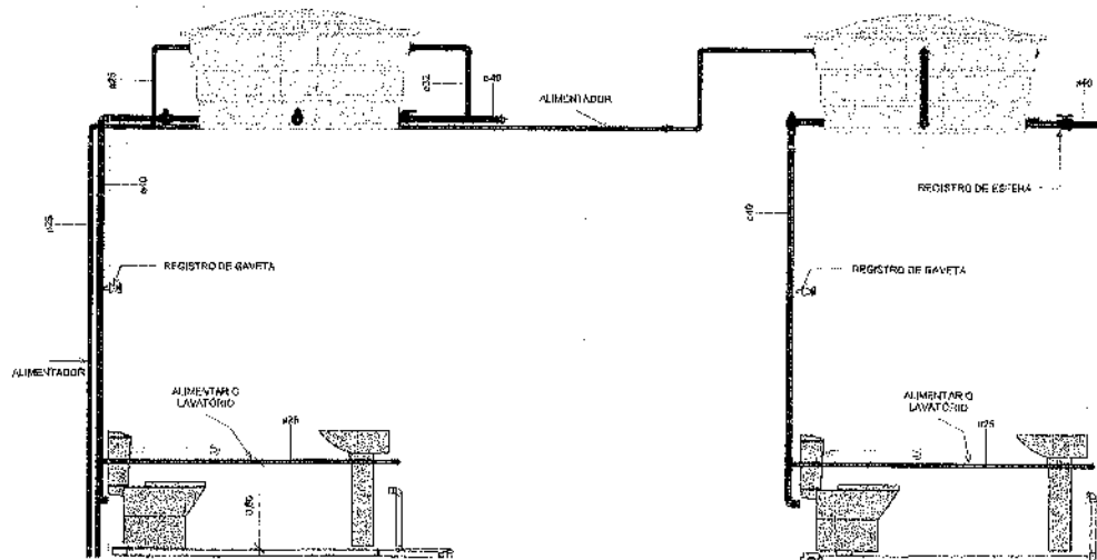
2 CORTE 02 1:20
