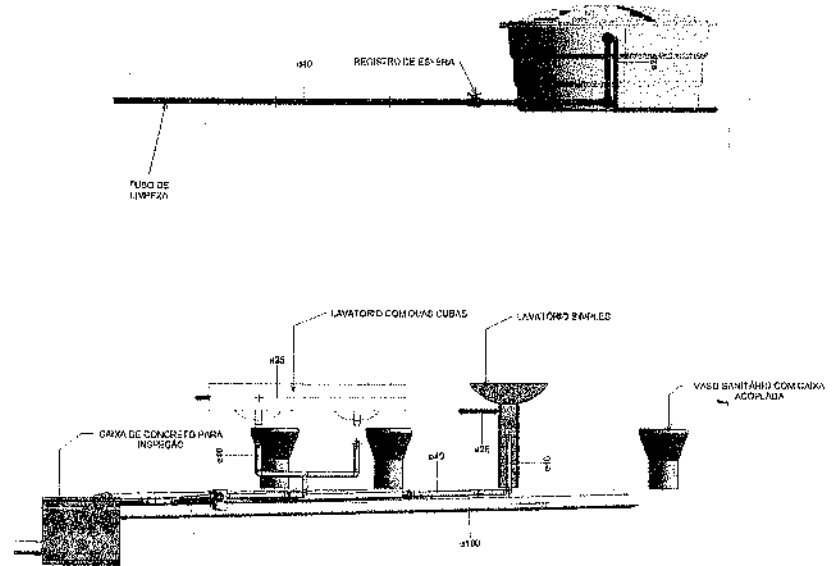
3 CORTE 03 1:20
