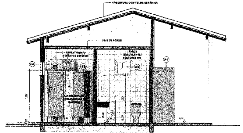
3 CORTE TRANSVERSAL DOS BANHEIROS 1:30
