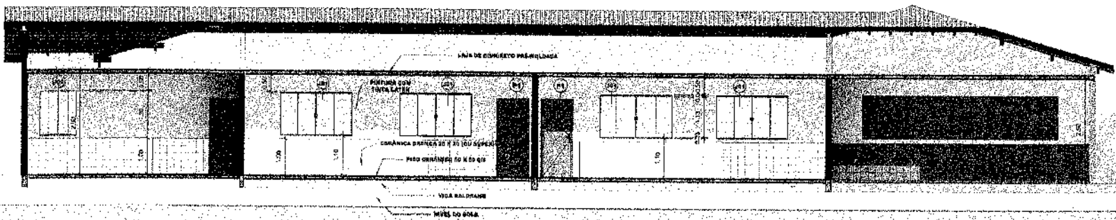
1 CORTE LONGITUDINAL SALAS 2 1:50
