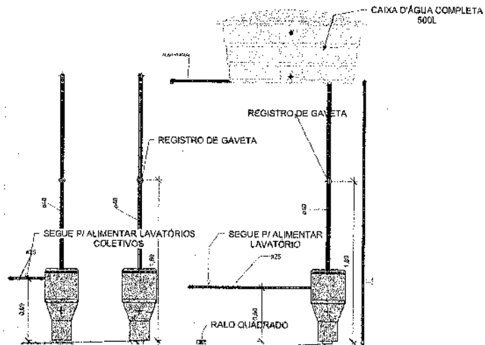
1 CORTE BAN. MASC 1:20
