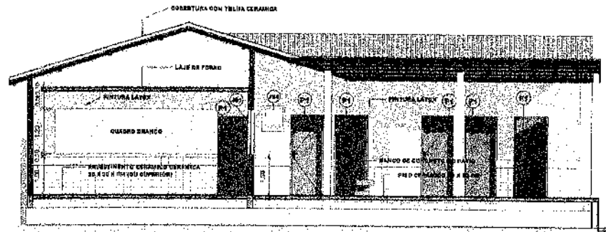
2 CORTE TRANSVERSAL SALAS AMPLIAÇÃO 1:50
