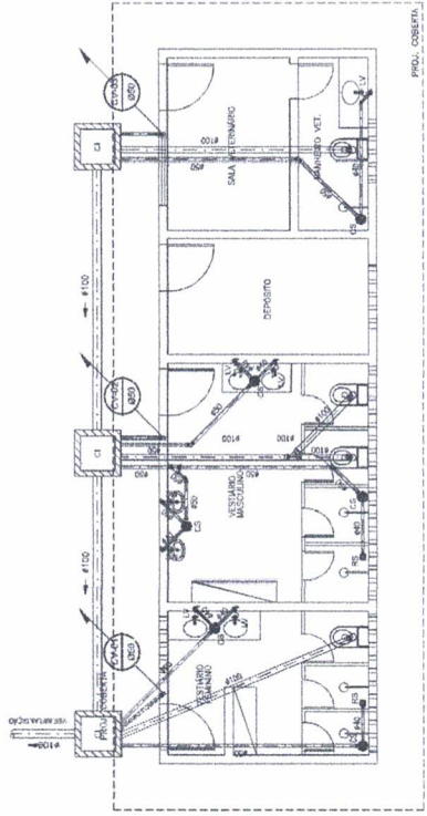
5 VESTIÁRIOS-ESGOTO SANITÁRIO esc.: 1:50
