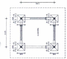
05 - LOCALIZAÇÃO DAS SAPATAS GUARITA
