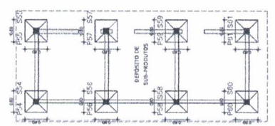
06 - LOCALIZAÇÃO DAS SAPATAS DEPÓSITO
