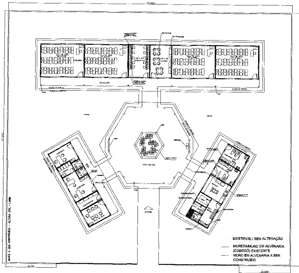
PLANTA BAIXA
