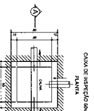
101 ESCALA 1:20
