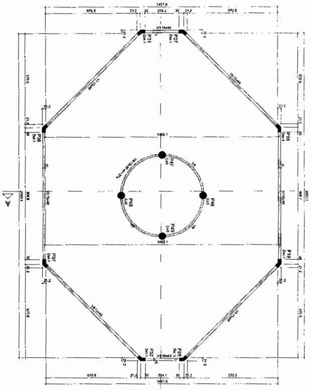
Forma do pavimento PÉ DIREITO - CENTRAL (Nível 715) escala 1:50
